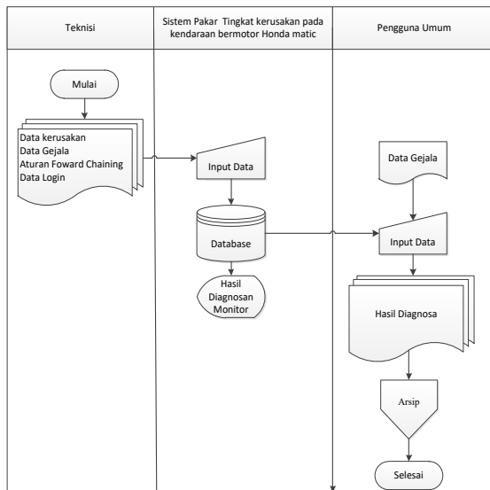
Alur dokumen
